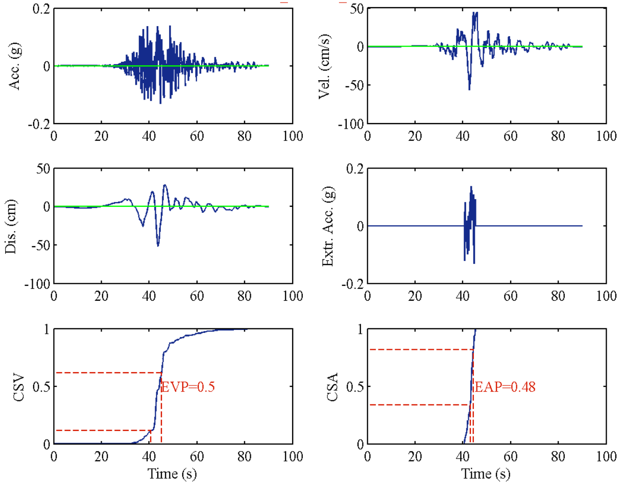
RSN1482_CHICHI_TCU039-N
