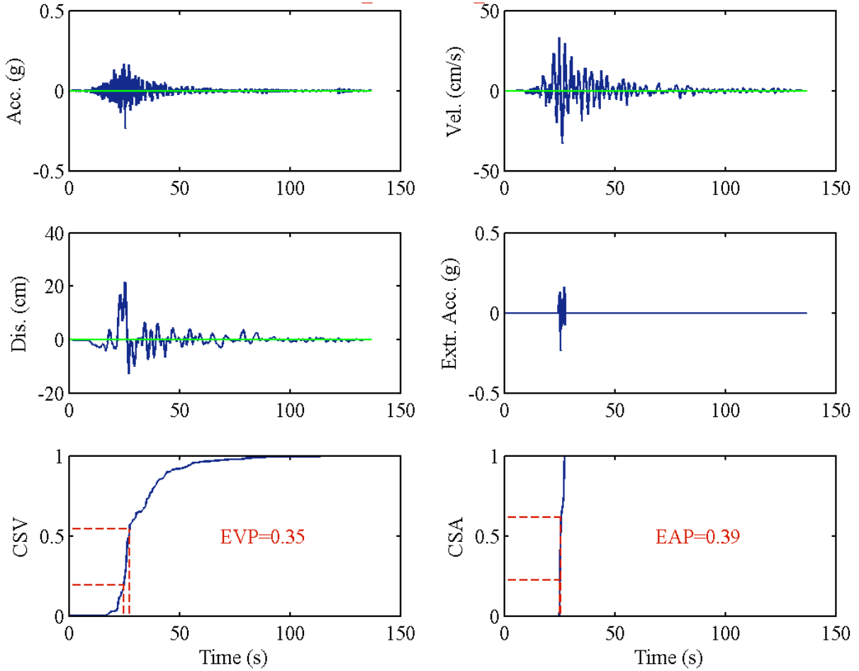
RSN6888_DARFIELD_CCCCN64E
