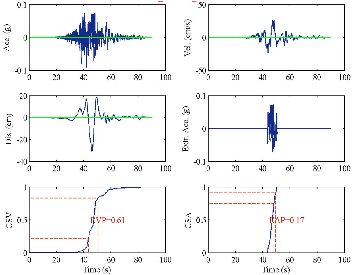
RSN1475_CHICHI_TCU026-N
