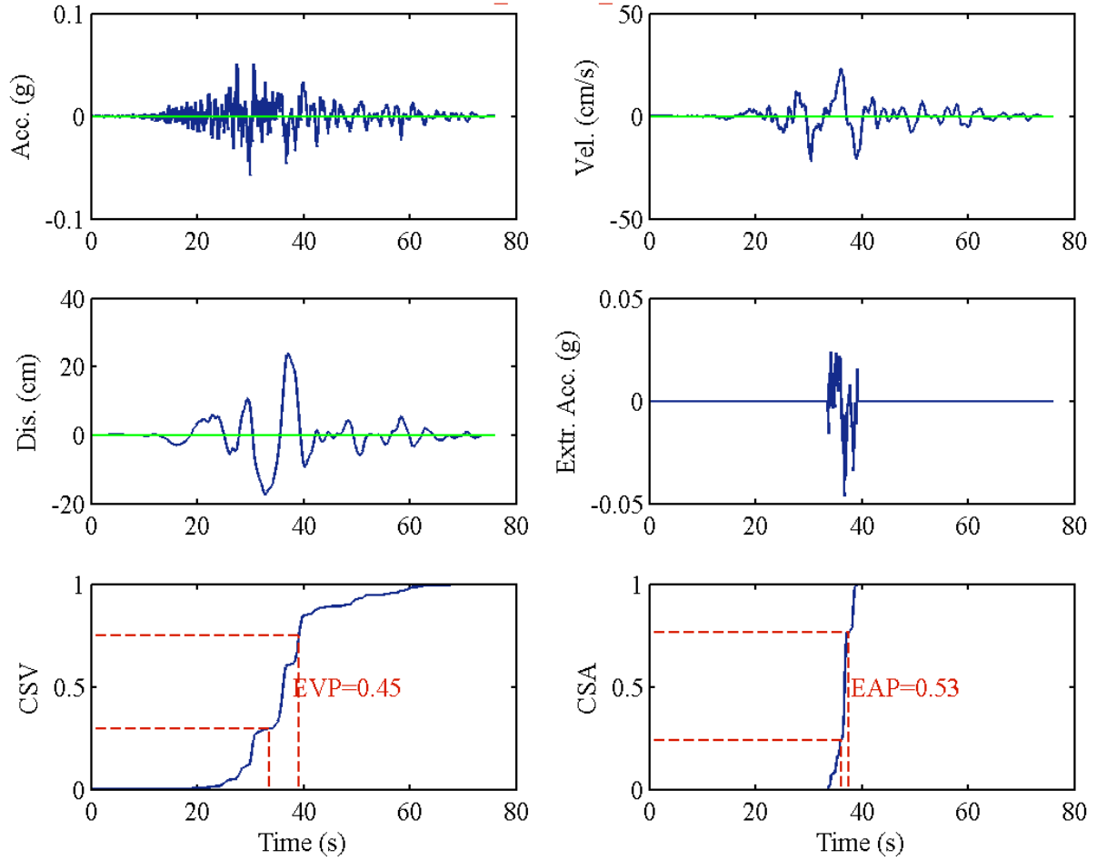
RSN1473_CHICHI_TCU018-N
