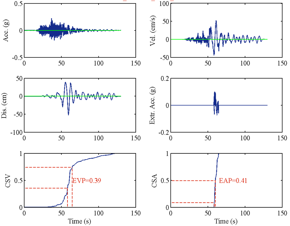
RSN5832_SIERRA_MEX_TAM090
