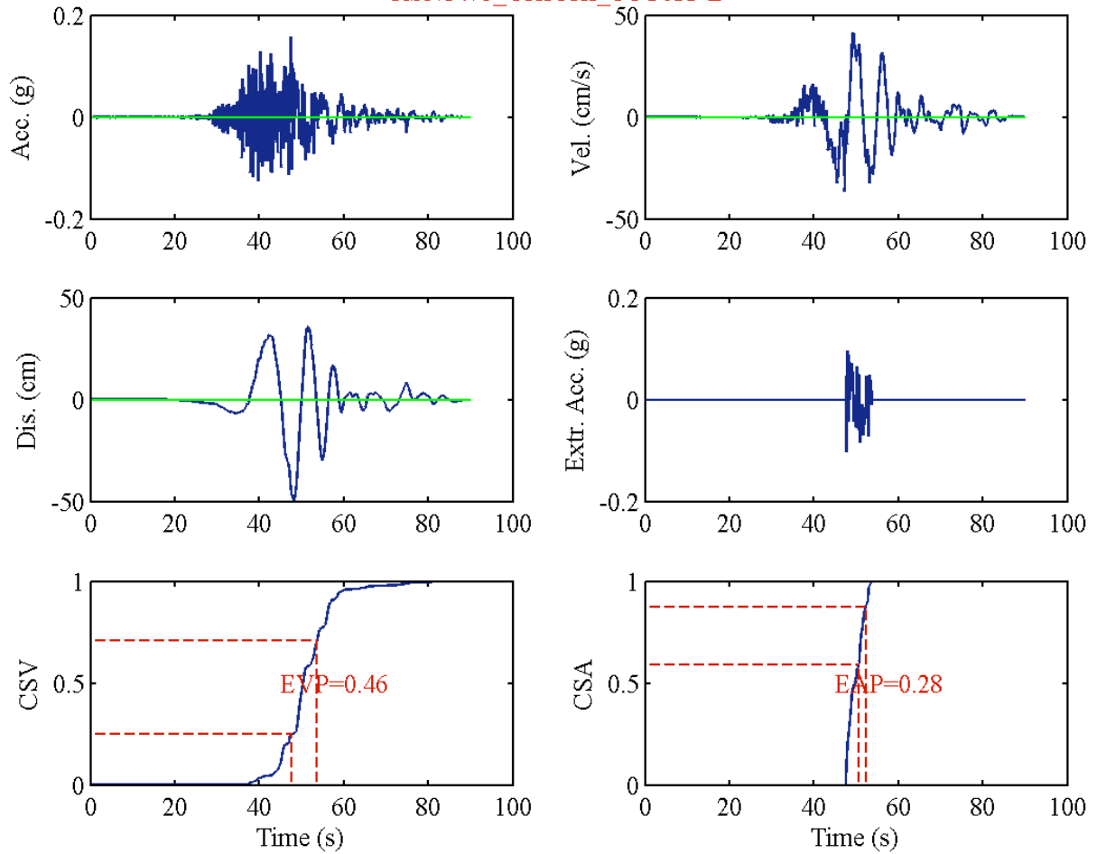
RSN1478_CHICHI_TCU033-E
