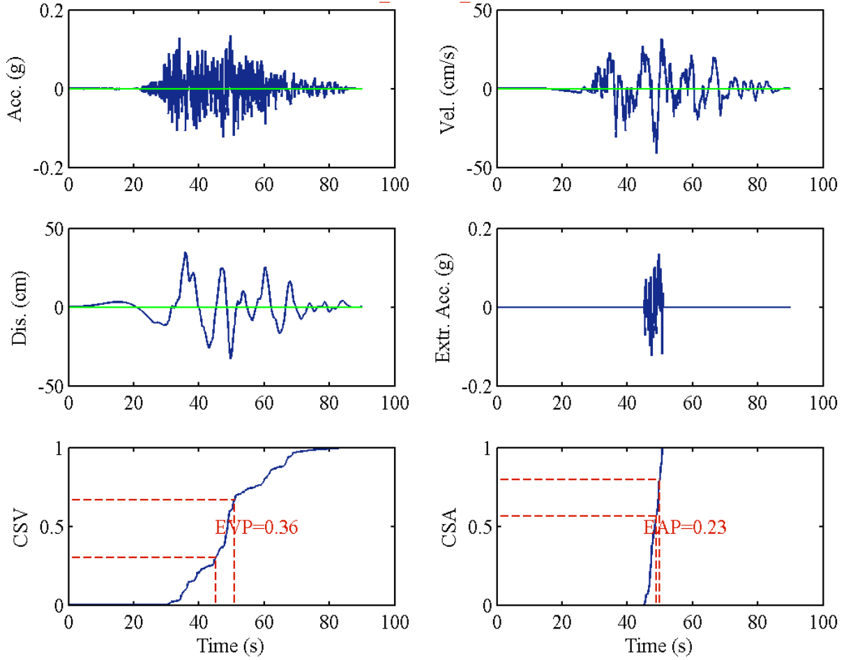
RSN1500_CHICHI_TCU061-E
