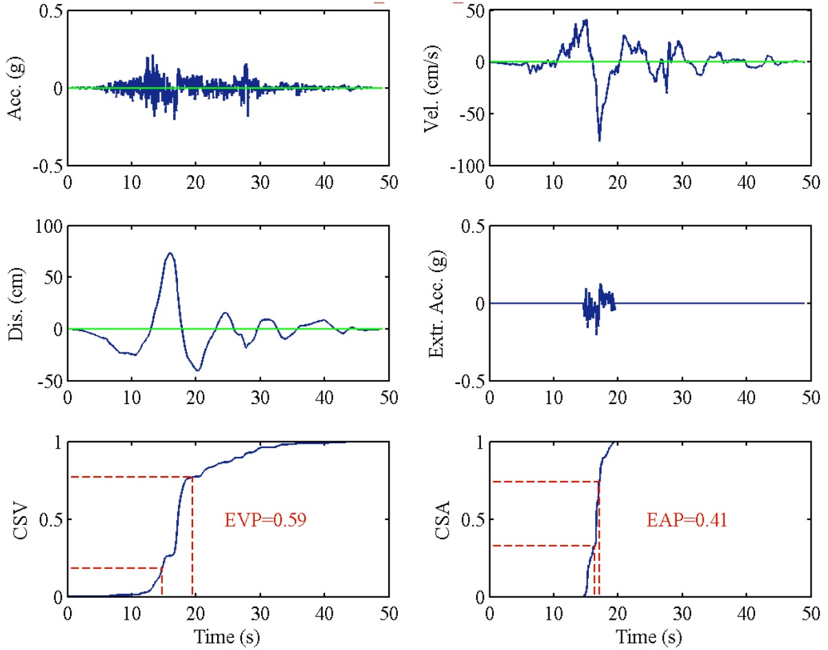
RSN1528_CHICHI_TCU101-E
