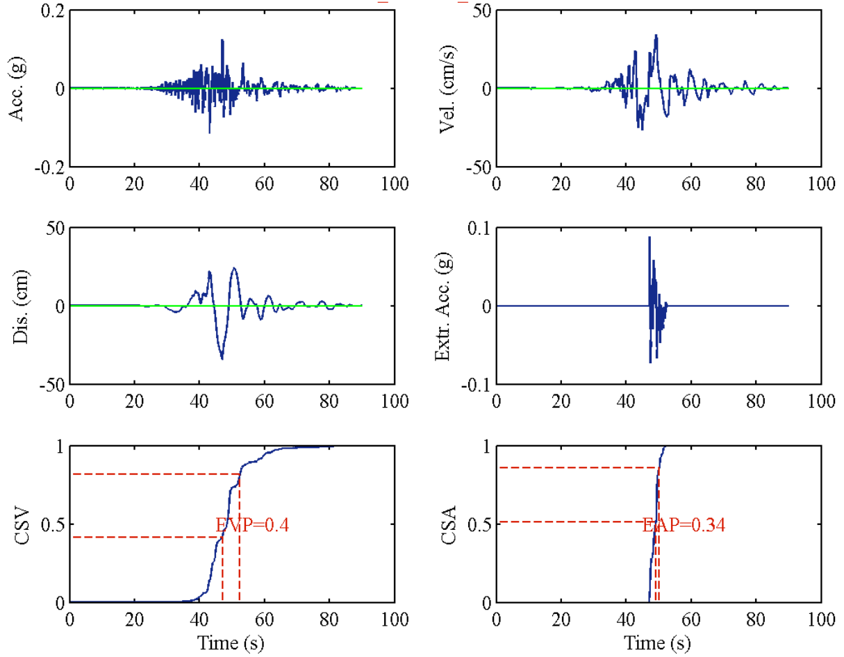
RSN1472_CHICHI_TCU017-N
